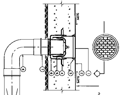
รูปที่ ๖ โถชำระแบบน้ำชำระพื้นห้องน้ำ
