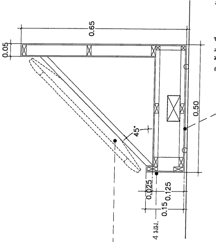
SECTION A-6 SCALE 1 : 15
