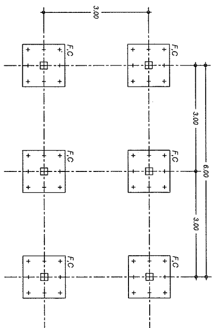
แผนผังฐานราก เสาตอม่อ
