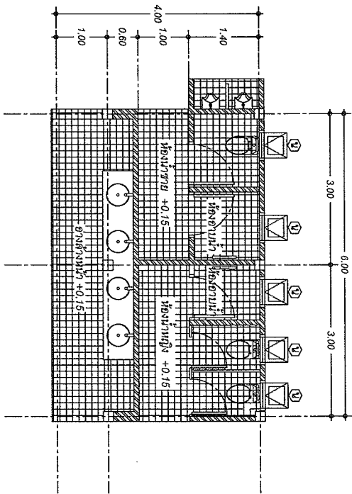
แปลนอาคาร 1 : 50
