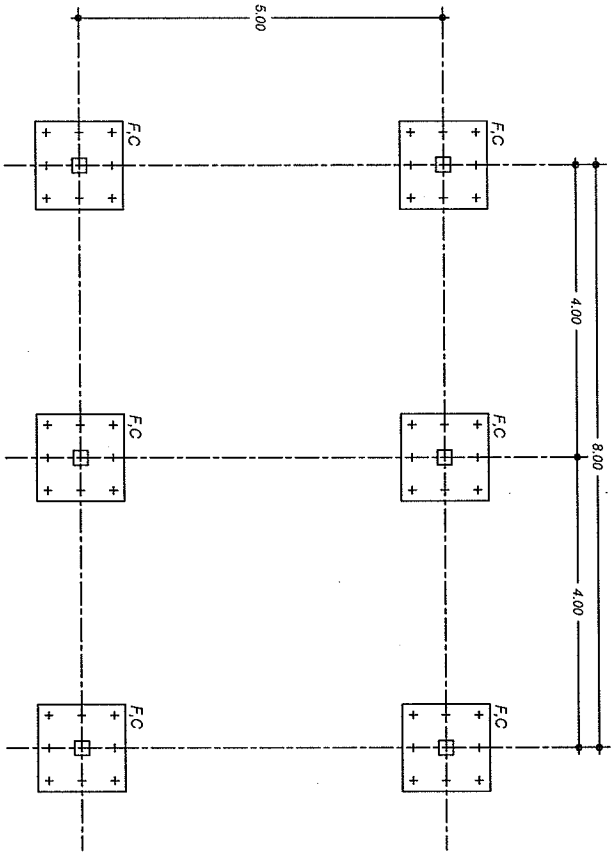
แผนผังเสาในโรงรถ
