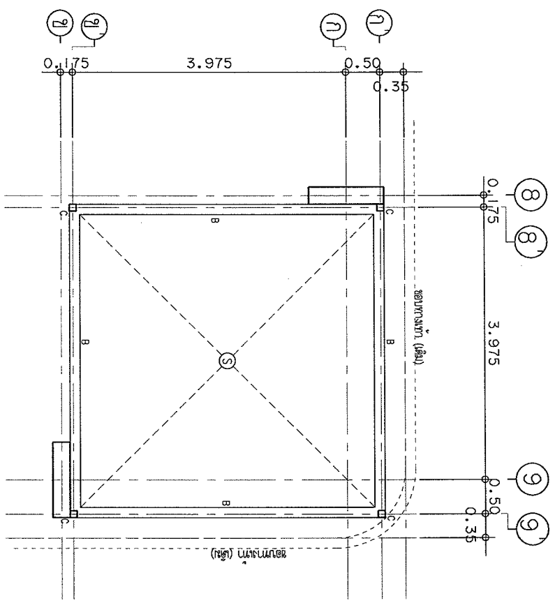
แปลนโครงสร้างคาน พื้น SCALE 1:50
