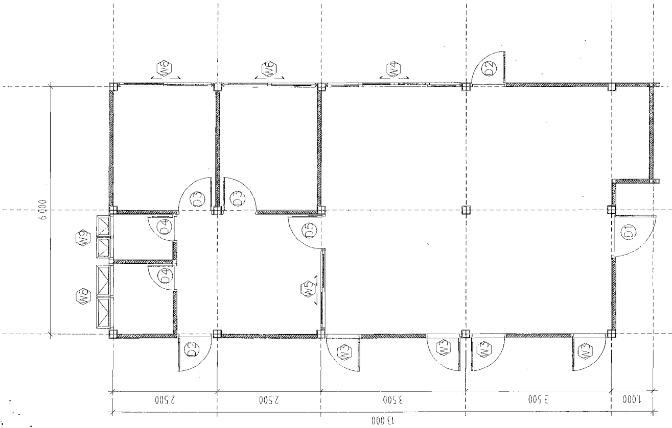
แบบแปลนชั้น1บ้านพัก ผอ. และ ผอ. มาตราส่วน 1/100
