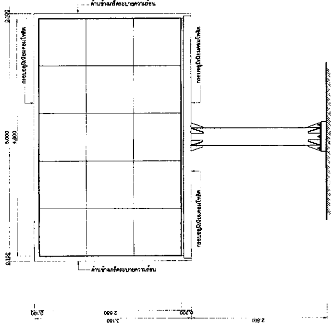
รูปตัดหน้า ขนาดย่อ 1:25
