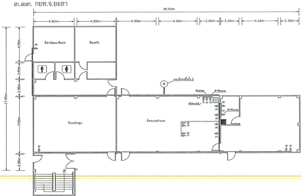
รูปแบบแปลน ชั้น ๑
