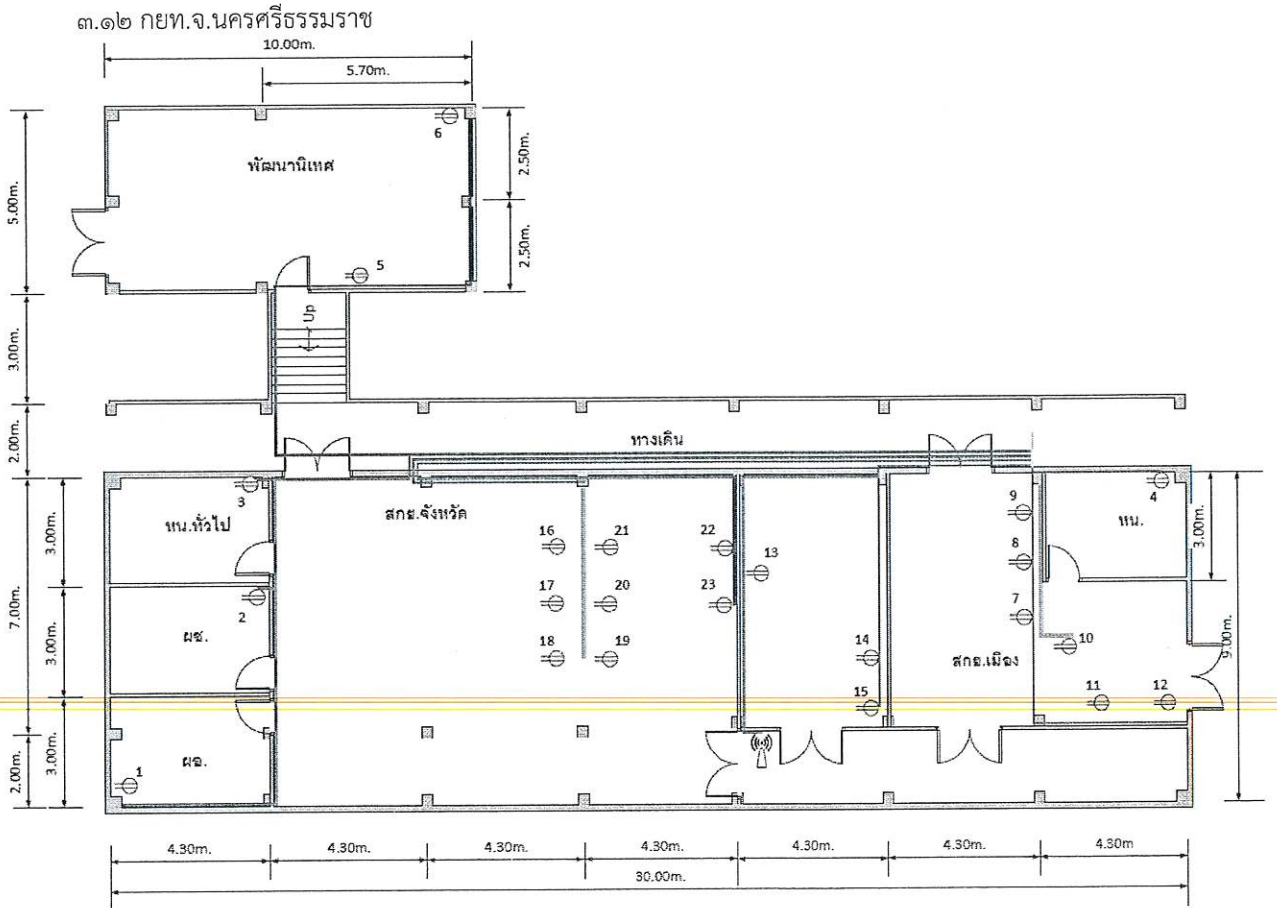
แบบแปลน ชั้น ๑
