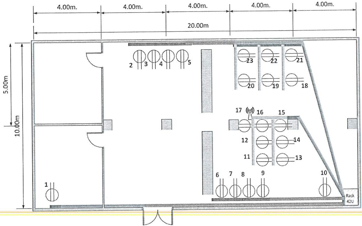
กยท. สาขาเมืองตรัง แบบแปลน ชั้น ๑
