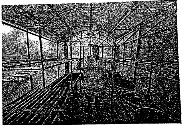
โรงอบยางพาราพลังงานแสงอาทิตย์ สำหรับใช้ในการอบยางแผ่นดิบ หลังการทำแผ่น โดยใช้พลังงานแสงอาทิตย์ทำให้ยางแผ่นแห้งเร็วขึ้น แม้ในช่วงที่ฝนตก แผ่นยางเหลืออยู่ สวย เป็นยางแผ่นดิบเกรดคุณภาพ อบได้ครั้งละ 800 แผ่น
